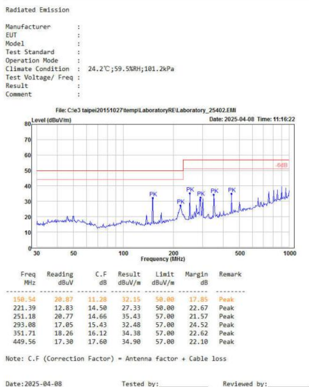
图 6-6 辐射测试水平方向
