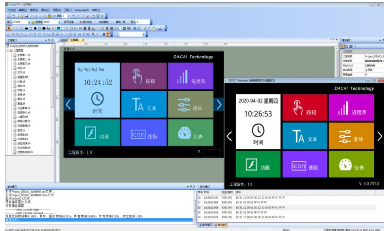
图 8-1 VisualTFT 主界面
