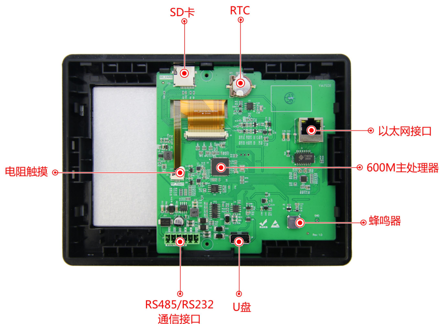
图 1-2 硬件配置图
