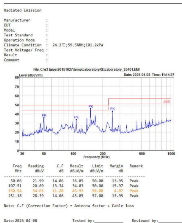
图 6-7 辐射测试垂直方向
