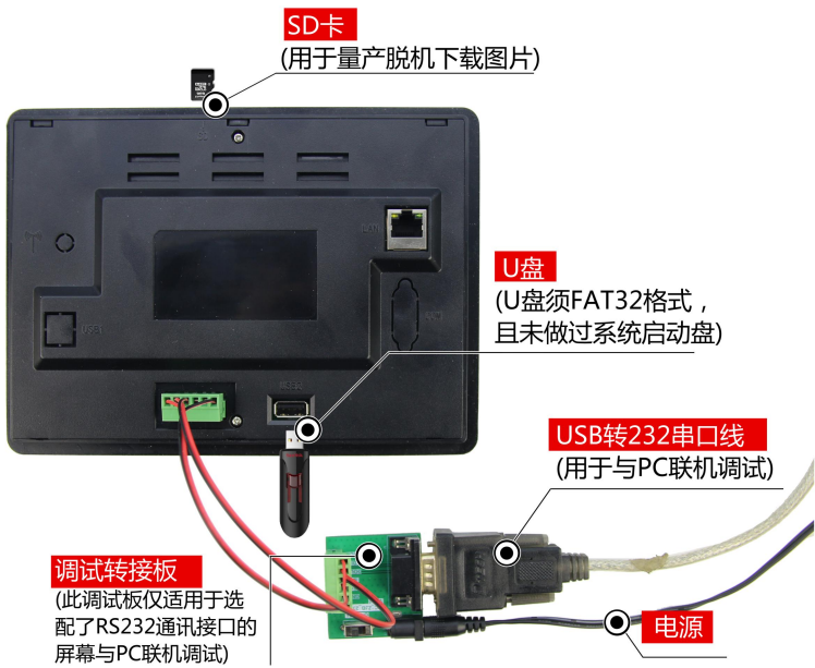
图 1-3 RS232 调试工具图
