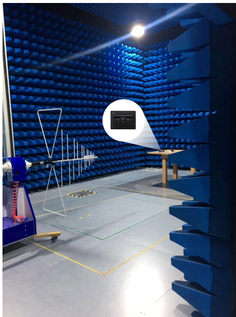
图 6-5 辐射测试图
