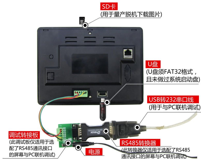
图 1-4 RS485 调试工具图
